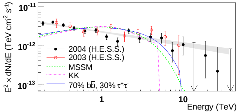
Abbildung 3.6: Die differentieller Spektrum der \gamma -Strahlungsquelle HESS J1745-290 aus Aharonian et al. (2006c). Die Punkte geben zeigen die von H.E.S.S. gemessenen Daten. Die drei Linien sind berechnete Spektren für verschiedene Modelle von Annihilation von dunkler Materie (auf die nicht näher eingegangen wird.)
