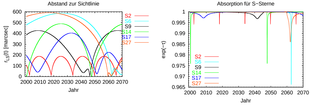
Abbildung 4.7: Links : Abstand zur Sichtlinie für S-Sterne. Rechts : Absorption e^{-\tau} für diese S-Sterne bei einer Energie von 200 GeV.
