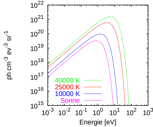
Abbildung 4.2: Photonendichte eines schwarzen Strahlers für verschiedene Temperaturen in \text{ph cm}^{-3} \text{eV}^{-1} \text{sr}^{-1} (doppelt-logarithmische Darstellung).
