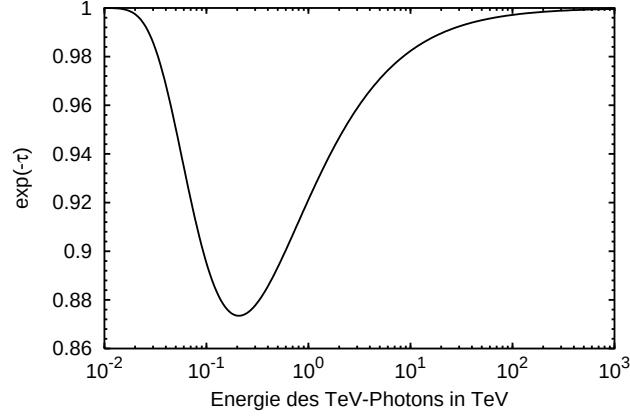
Abbildung 4.6: Energieabhängigkeit der Absorption e^{-\tau} für einen Stern mit T_{\text{eff}} = 25000 \text{ K} , R_* = 10.7 R_{\odot} und einen festen Abstand von r_{\text{LS}} = 0.5 \text{ mas} .
