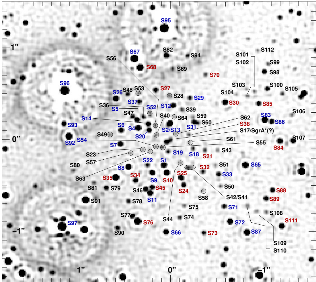
Abbildung 3.8: Das galaktische Zentrum im nahen Infrarot (Gillessen et al. 2008). Das Bild zeigt eine Aufnahme des NaCo-Detektorsystems (H-Band), in der Mitte befindet sich die Radioquelle Sgr A* . Die Farben der Bezeichnungen der Sterne geben den Spektraltyp an (blau: früher Sterntyp, rot: später Sternyp, schwarz: unsicher).
