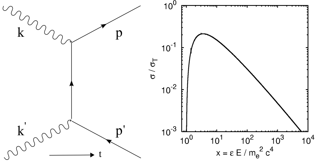
Abbildung 4.1: Links: Feynmangraph der Paarerzeugungsreaktion. k und k' bezeichnen die Vierervektoren der Photonen, p und p' sind die Vierervektoren des Elektrons und des Positrons. Rechts: Über alle Winkel integrierter (totaler) Wirkungsquerschnitt der Paarerzeugung in doppelt-logarithmischer Darstellung.
